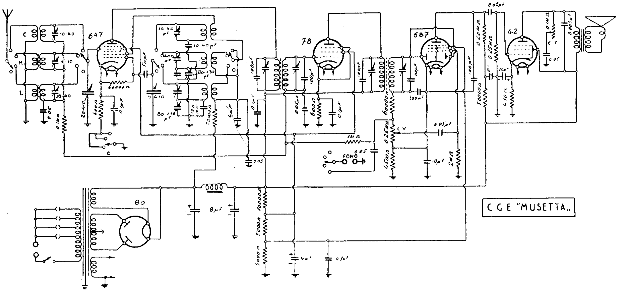
COMPAGNIA GENERALE DI ELETTRICITÀ. — Mod. « Musetta ». - Produzione 1937. - Media frequenza: 459 kHz.
